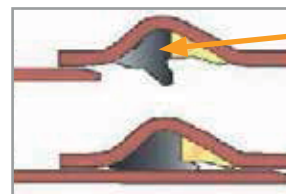
SEWER-Lock-Dichtring/ POWER-Lock-Dichtring ähnlich
